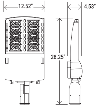
PT-AL1-150W-5K / PT-AL1-200W-5K
