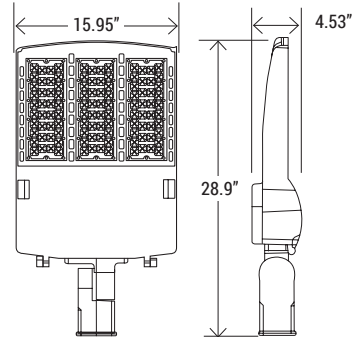
PT-AL1-240W-5K / PT-AL1-300W-5K
